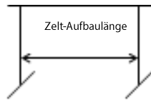
Form II für Teilzelt - mittig eingezogen, erforderlich: zwei Andrückstangen
